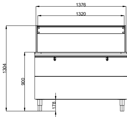
Fronte
